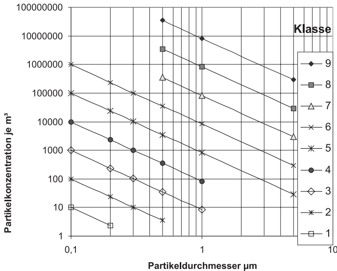
Bild F2-30 Reinraumklassen nach ISO 14644 [F-32]
